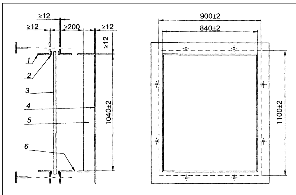
1 - зажимающая рама; 2 - резиновая полоса; 3 - испытываемый образец; 4 - жесткая стальная рама; 5 - мягкая прокладка; 6 - отверстия
