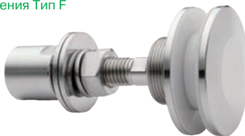
Узел крепления Тип F
